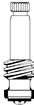
42045 Stem RH 42046 Stem LH
